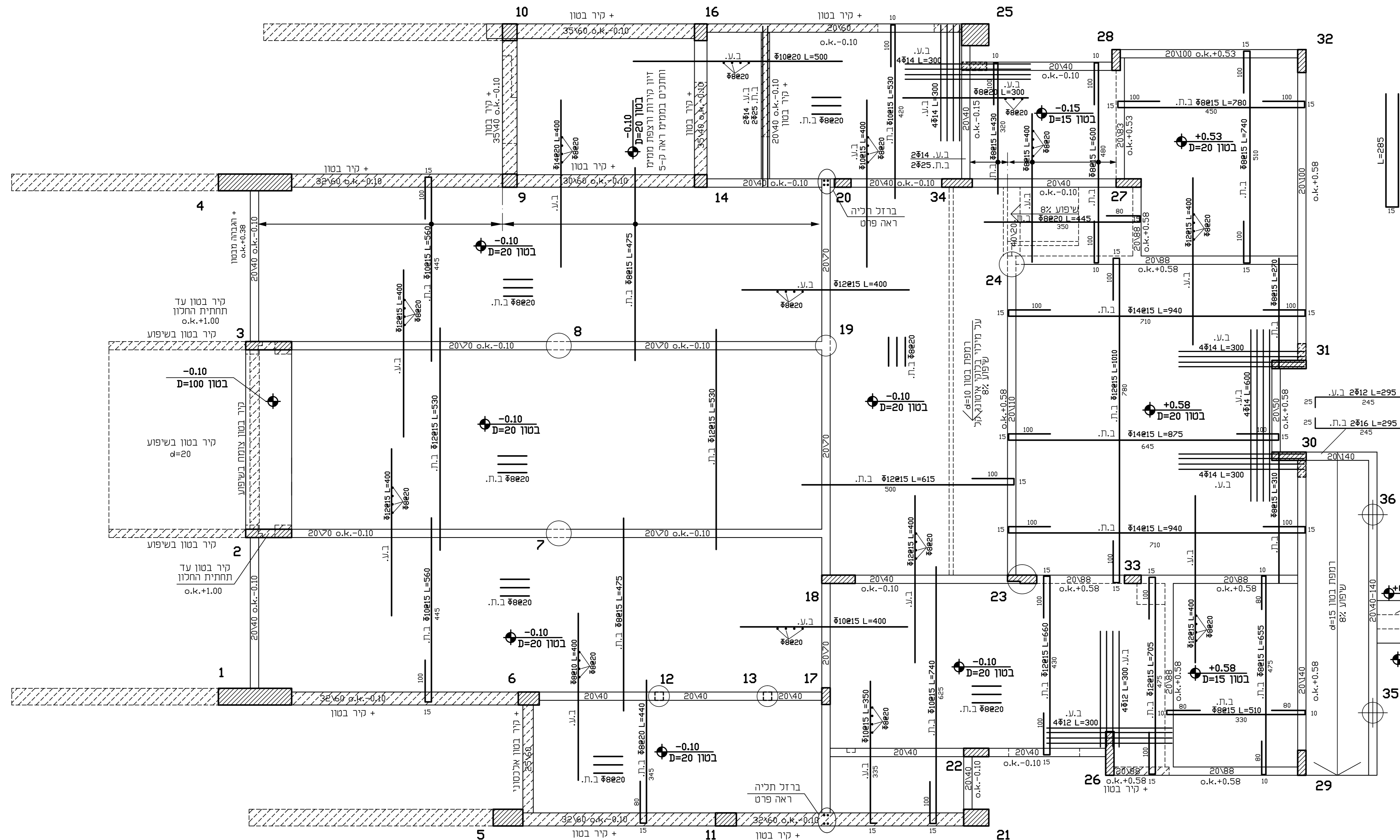
תכנית רצפה 1:50
