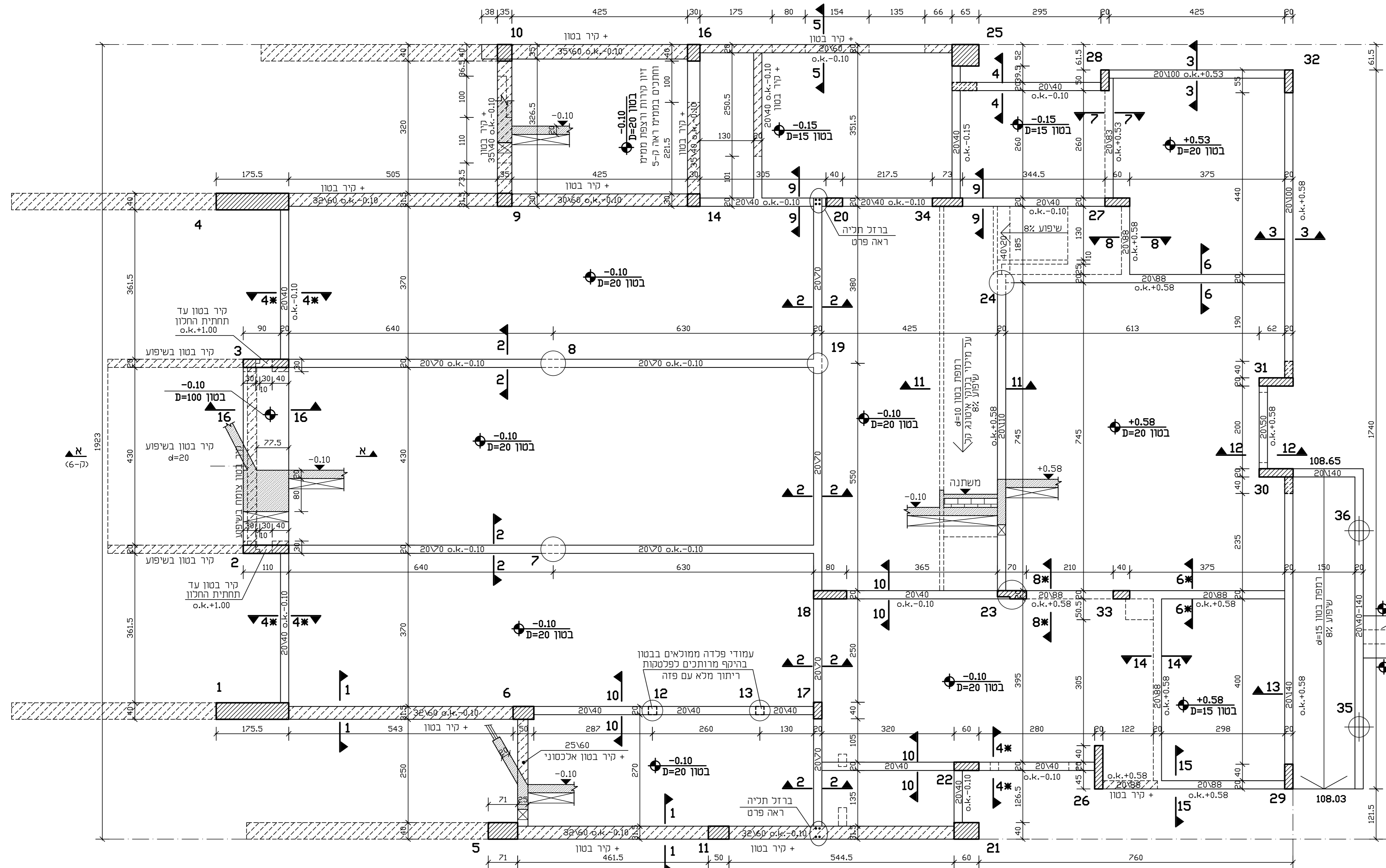
תכנית רצפה 1:50
