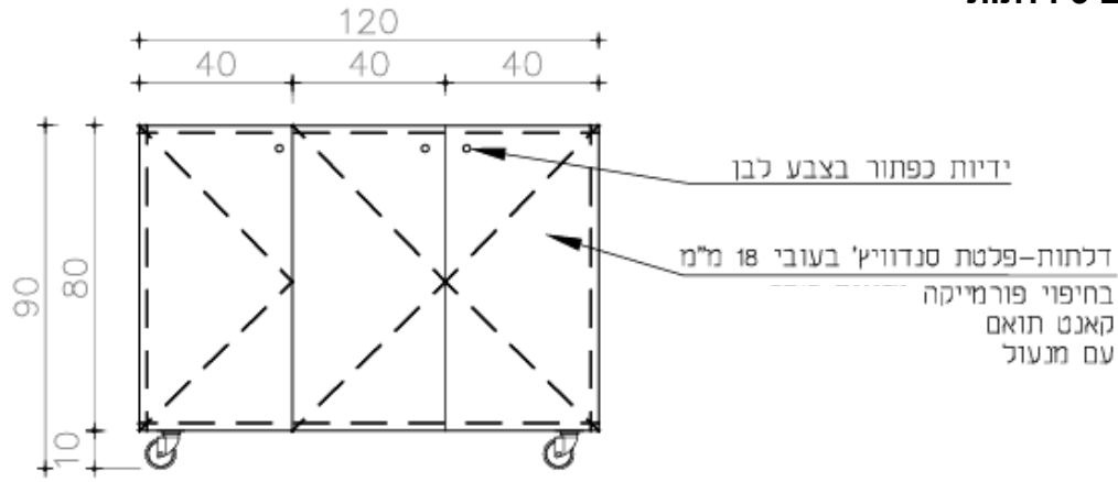
חזית 1
