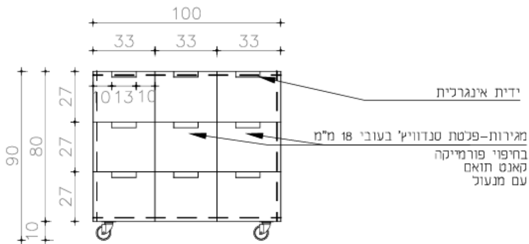
חזית 1
