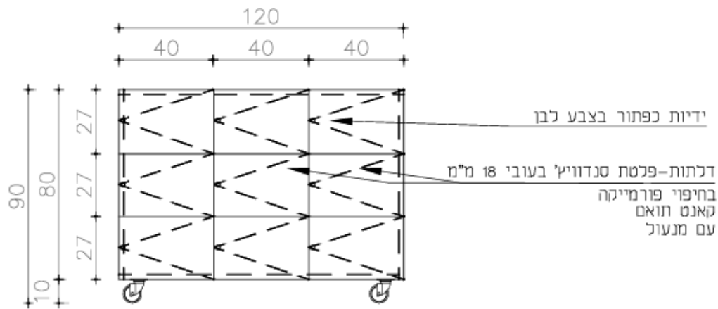
חזית 1
