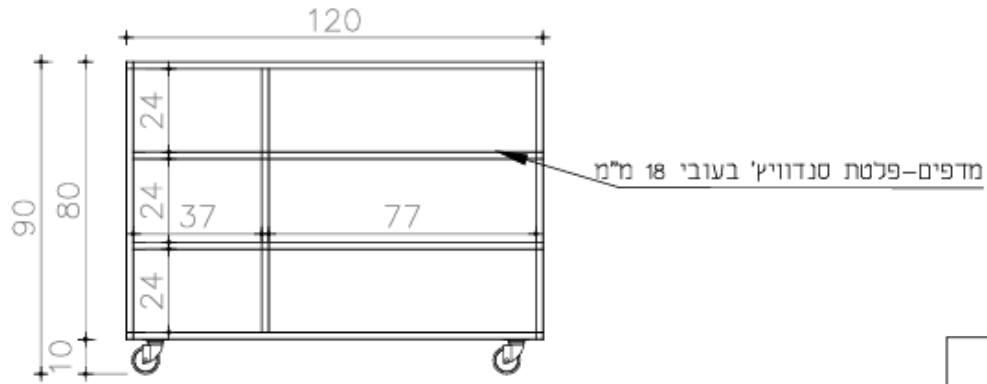
חלוקה פנימית
